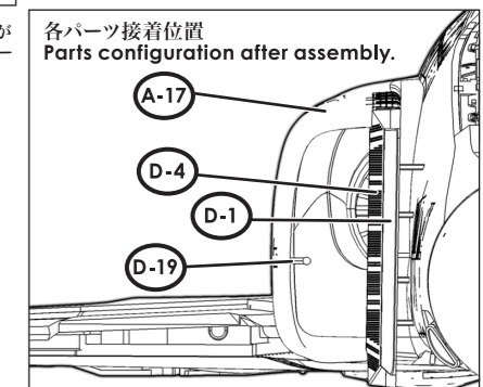
正面図 / Front View
