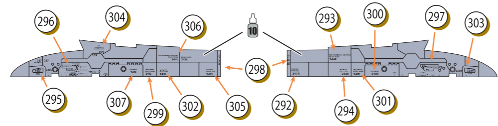
内側パイロン左側 (パーツR2/3) /Inner wing pylon - left (Parts R2/3)
