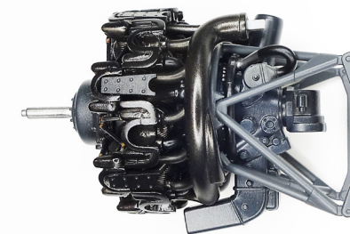
左側面写真 / Left Side View
