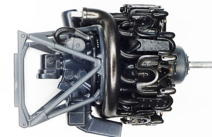
右側面写真 / Right Side View
