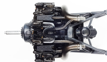
上面写真 / Top View
