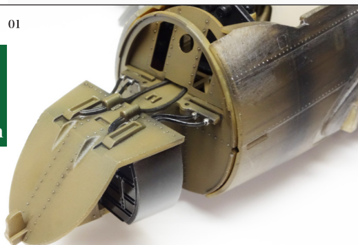
キ45改甲 Ki-45 Kai Ko
