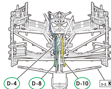
背面図 / Rear View
