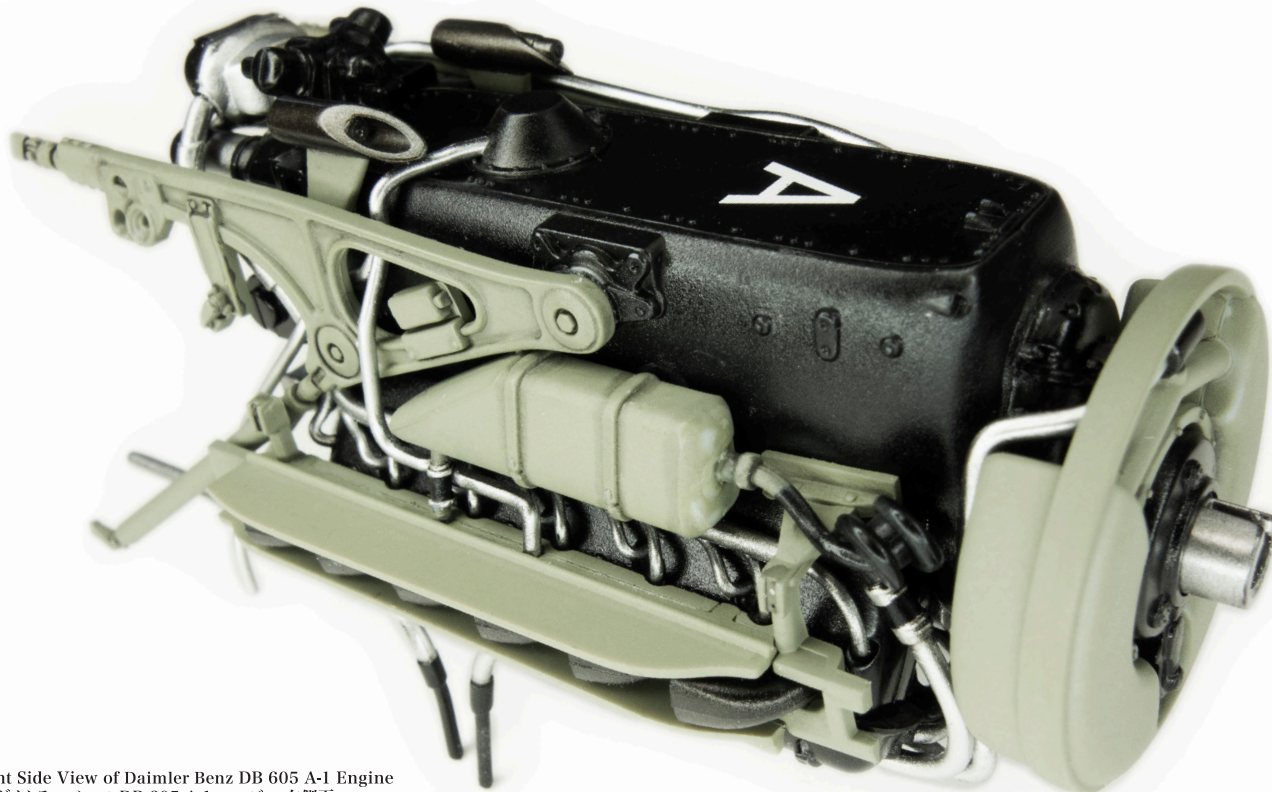
Right Side View of Daimler Benz DB 605 A-1 Engine / ダイムラーベンツ DB 605 A-1 エンジン 右側面
