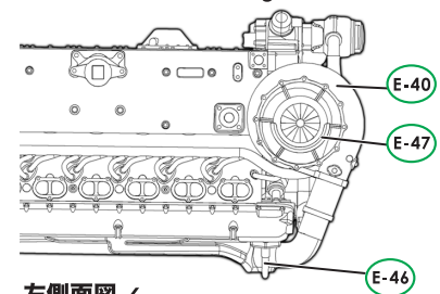
左側面図 / Left Side View
