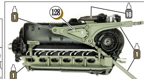
左側面図 / Left Side View
