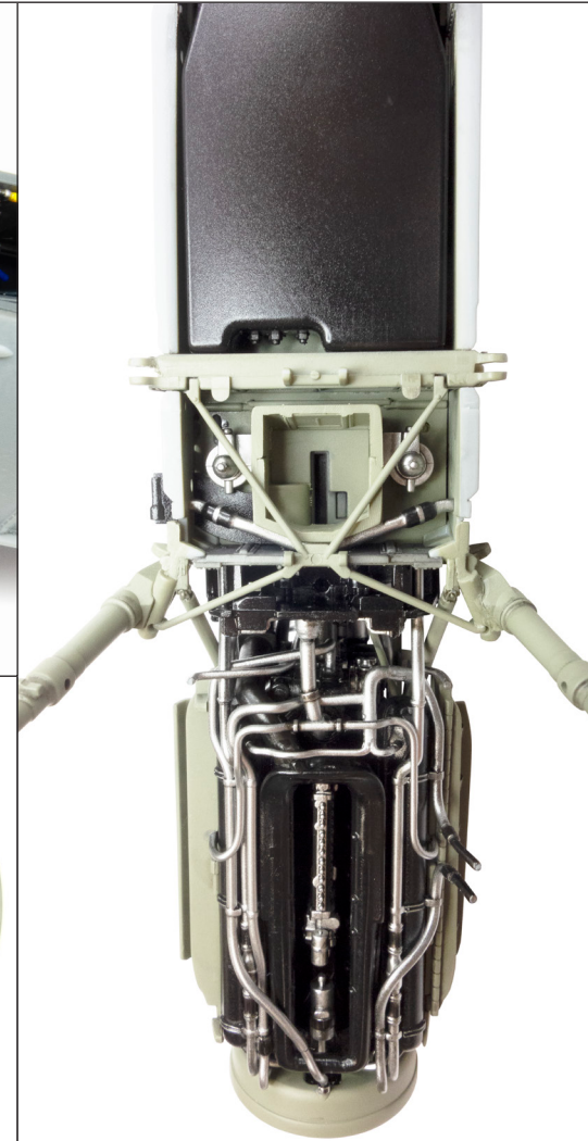
Bottom View of Fuselage ／ 胴体 下面
