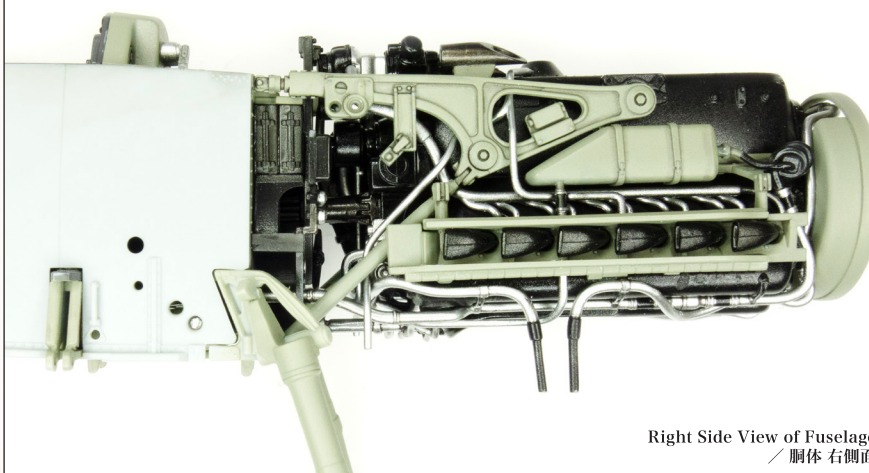
Left Side View of Fuselage ／ 胴体 左側面
