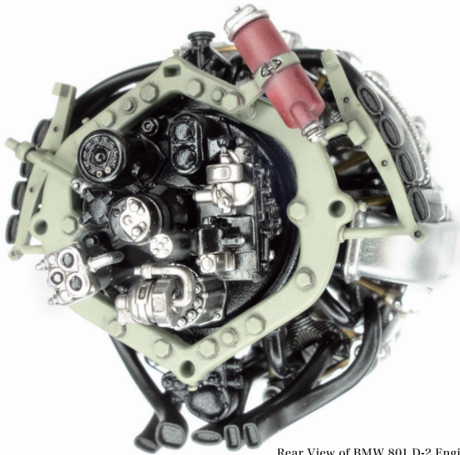
Rear View of BMW 801 D-2 Engine ／ BMW 801 D-2 エンジン 背面
