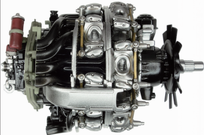
Right Side View of BMW 801 D-2 Engine ／ BMW 801 D-2 エンジン 右側面
