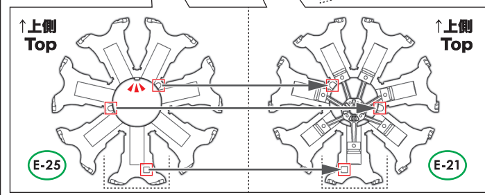
前列シリンダーブロック Front Cylinder Block
