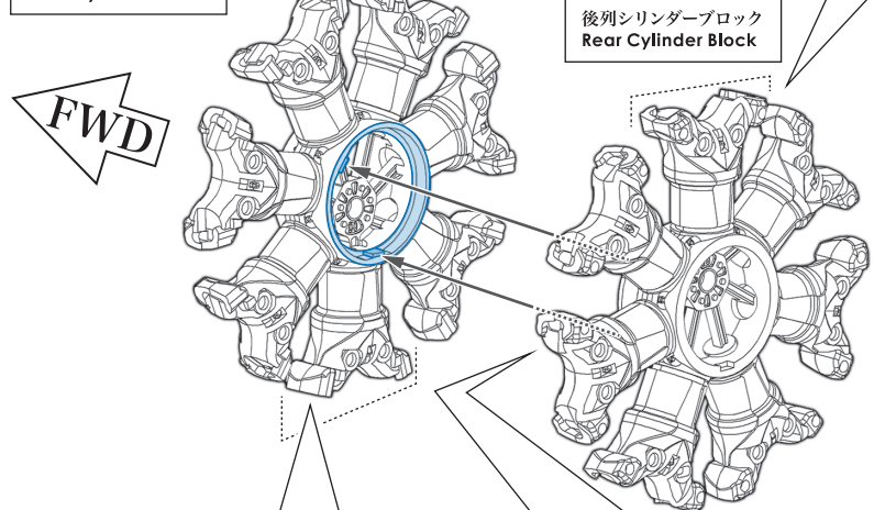
前列シリンダーブロック Front Cylinder Block
