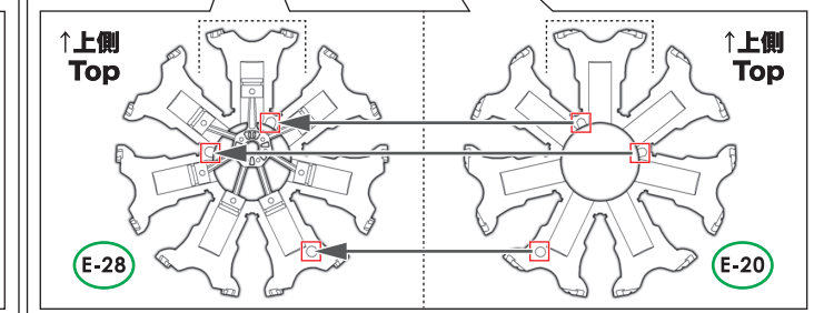
後列シリンダーブロック Rear Cylinder Block
