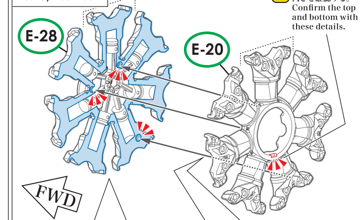
後列シリンダーブロック Rear Cylinder Block
