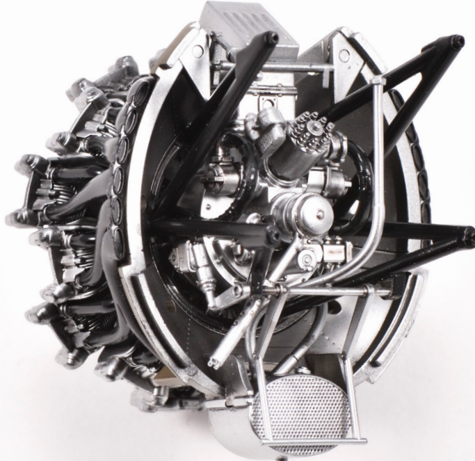
Rear View of Ha-112-II Engine / ハ 112-II 発動機 背面
