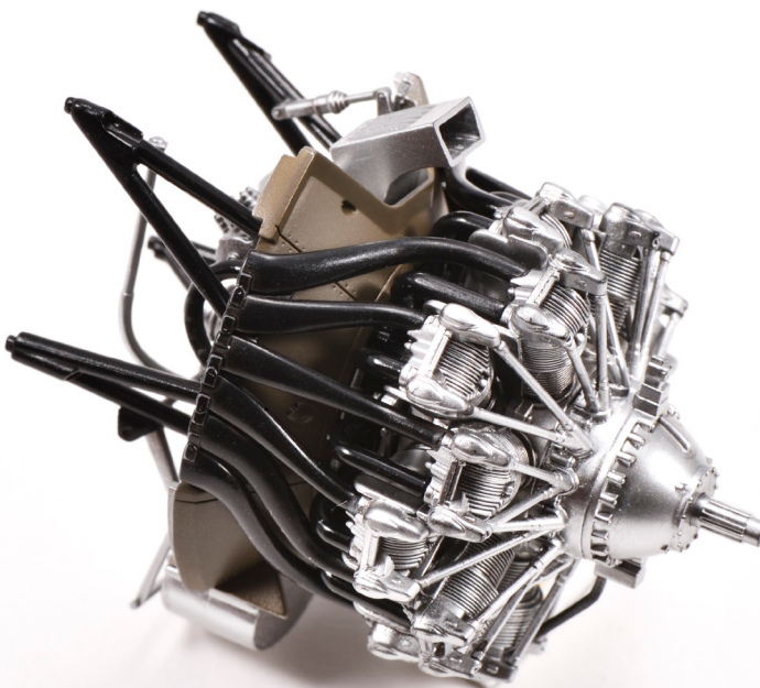
Right Side View of Ha-112-II Engine / ハ 112-II 発動機 右側面
