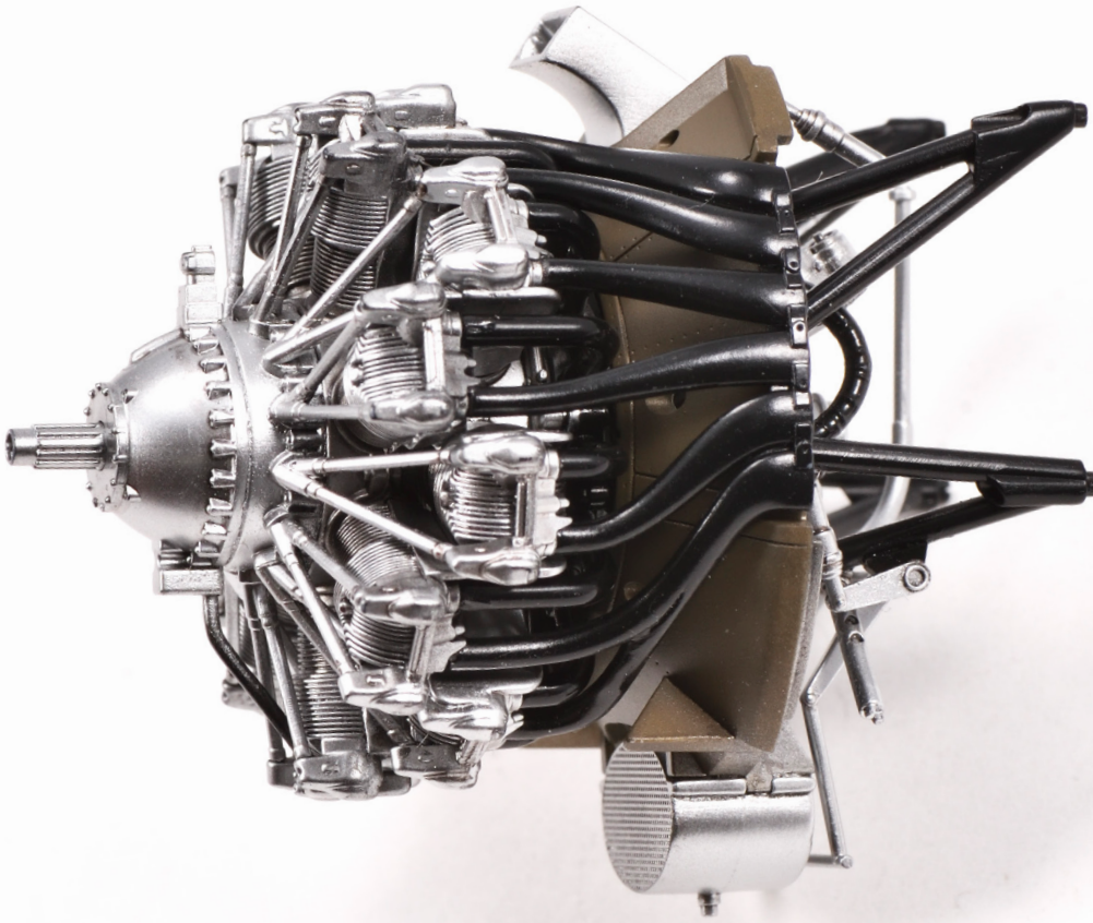
Left Side View of Ha-112-II Engine / ハ 112-II 発動機 左側面
