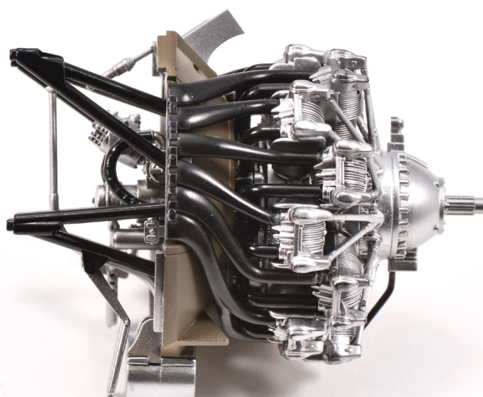
右側面写真 / Right Side View
