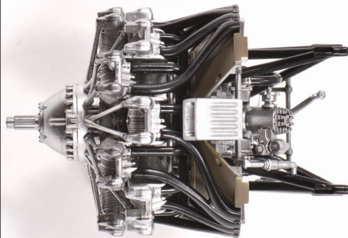
上面写真 / Top View
