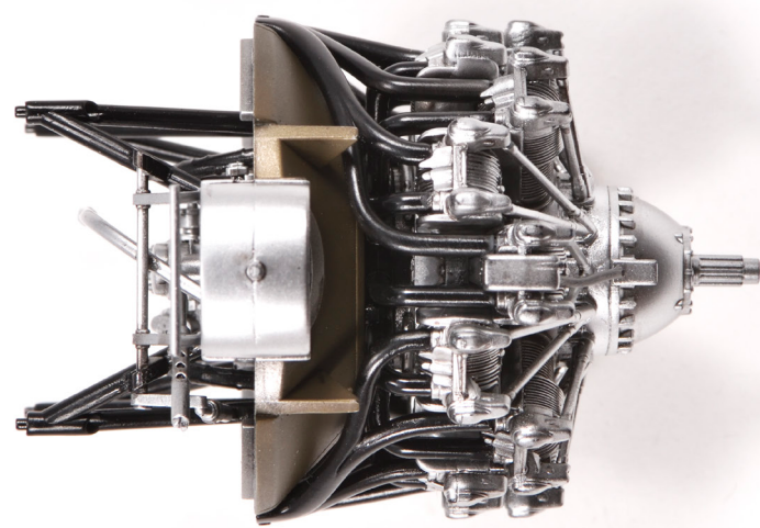
下面写真 / Bottom View
