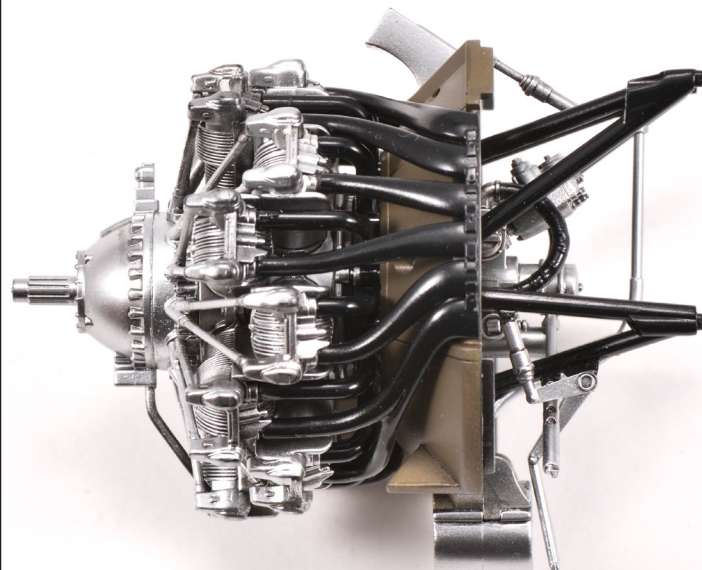
左側面写真 / Left Side View
